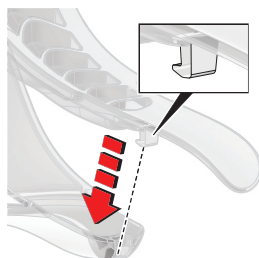
Háček konektoru
